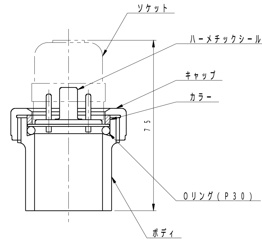
ハーメチックシール組立図
